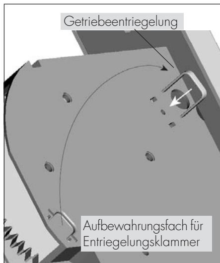
Rollotron® Pro comfort DuoFern® (Artikel-Nr. 9800)
